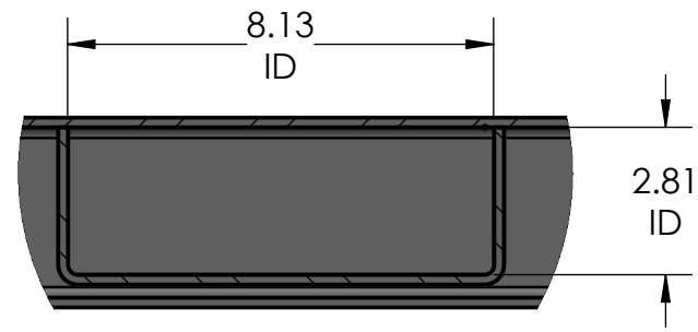
SECTION A-A SCALE 1 : 4
